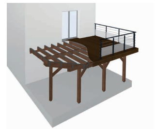
Stelzenkonstruktion (hohe Aufbauhöhe)
