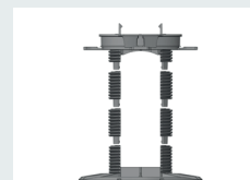
Basismodell mit 3 Paar Aufsätzen 146 - 190 mm
