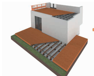
Auf stabilem Boden (Schotter)
