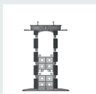
Basismodell mit 4 Paar Aufsätzen + 2 Versteifungen 200 - 235 mm
